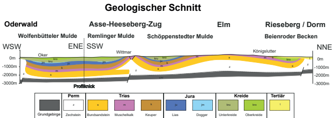
Geologischer Schnitt durch das Braunschweiger Land mit Elm und Asse
