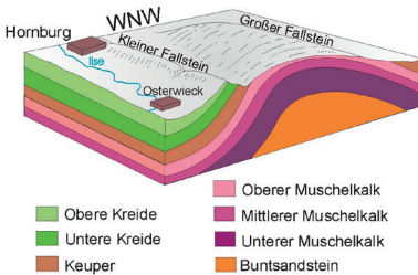
Die Aufwölbung der Fallstein-Struktur
